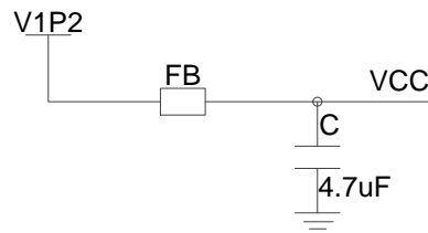
图 2 VCC 核电压输入端噪声处理
