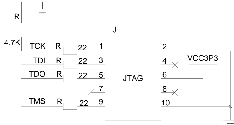
图 3 JTAG 电路参考
